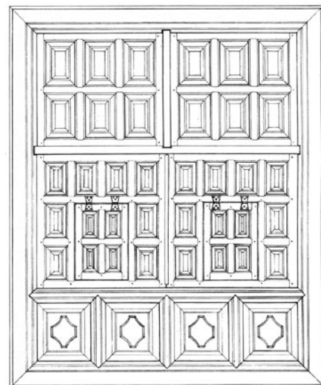
Ventana de Cuarterones
